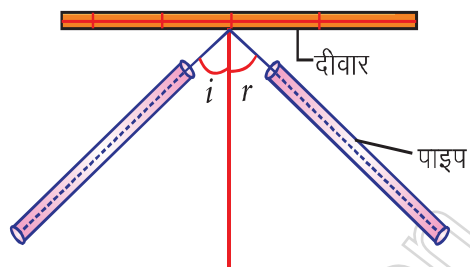
ध्वनि का परावर्तन
